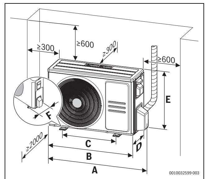
Bild 5 Abmessungen Außeneinheit
