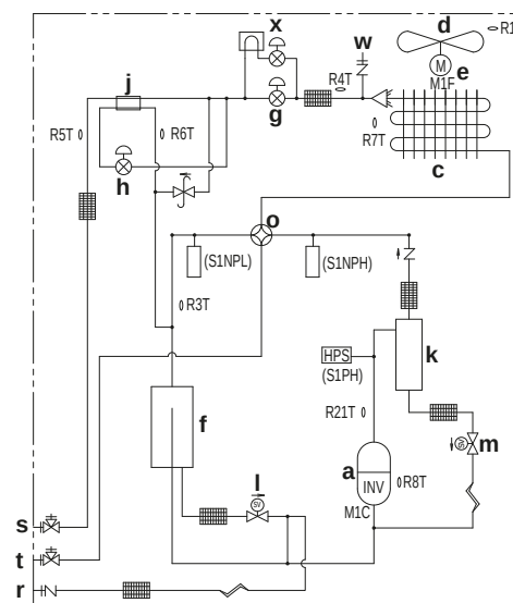
Rohrleitungsplan: RXYQ8~12
