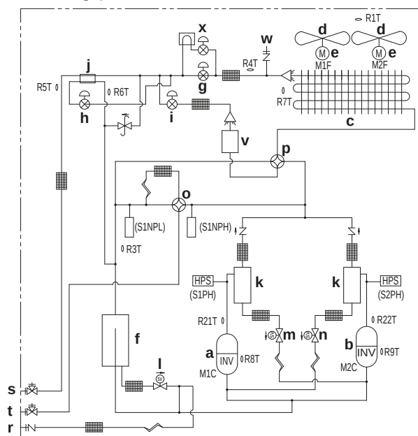
Rohrleitungsplan: RYYQ14~20
