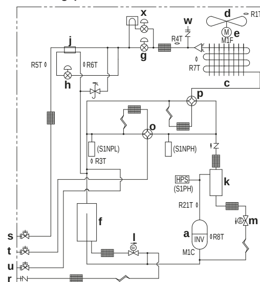
Rohrleitungsplan: RYMQ14~20
