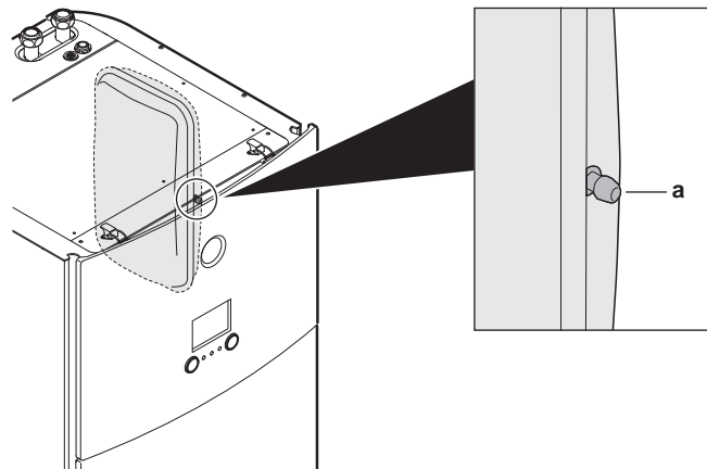
a Schrader-Ventil
