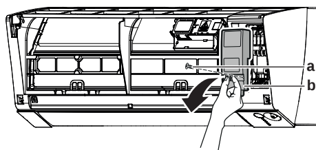
a Schraube von Wartungsblende b Wartungsblende
