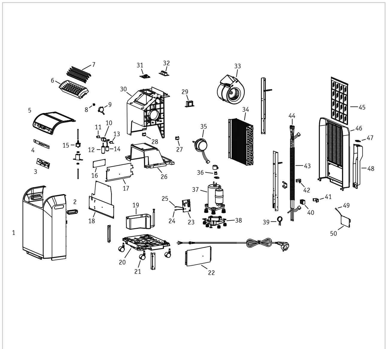
Abb. 19: Explosionszeichnung Innengerät
