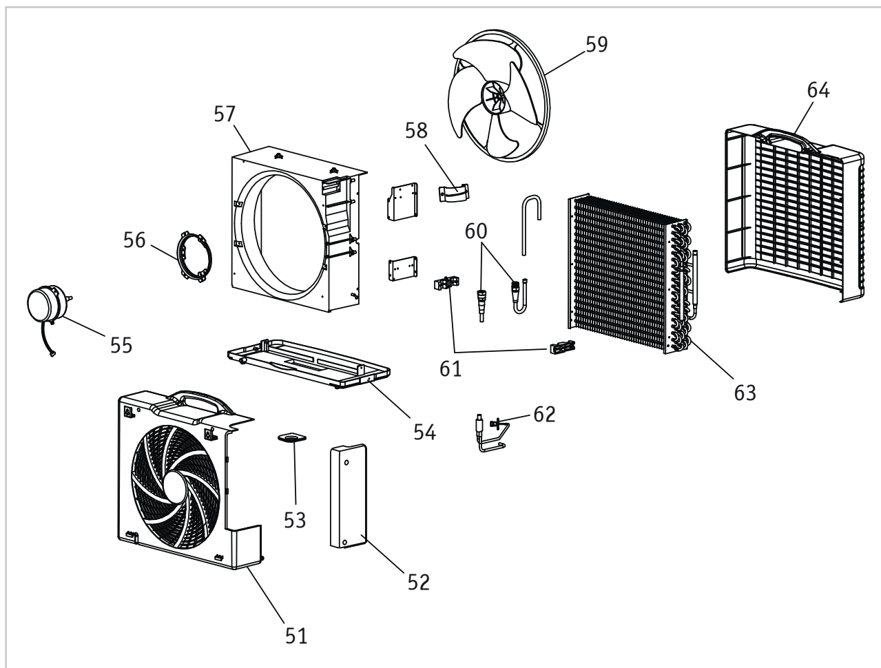
Abb. 20: Explosionszeichnung Außenteil
