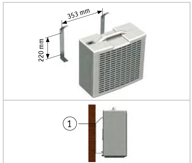
Abb. 9: Abstände Montagehalterung
