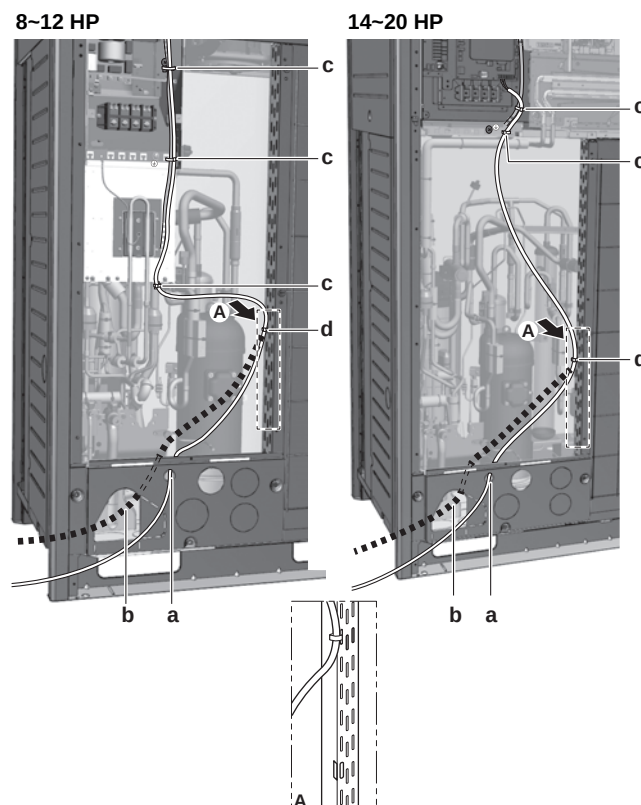
a Übertragungskabel (Möglichkeit 1) (a)
