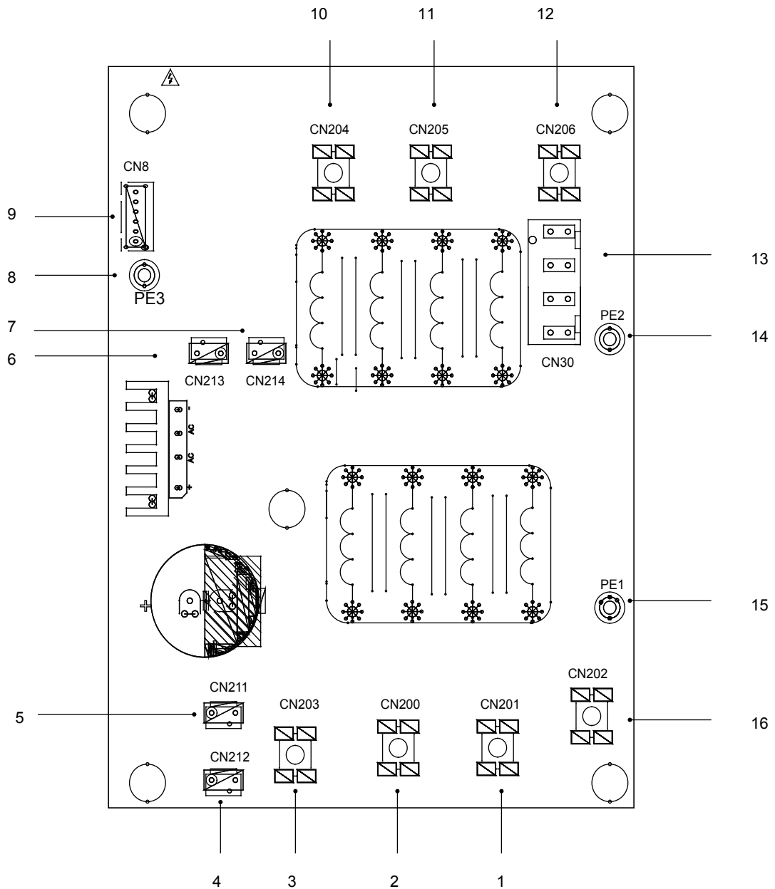
Leiterplatte C 3-phasig 12/14/16kW
