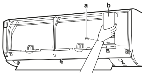
a Schraube von Wartungsblende
