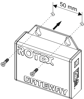
Bild 2: Wandmontage
